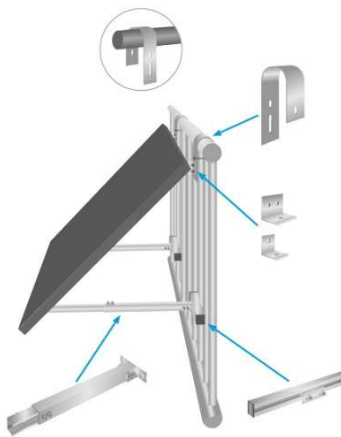
Gitter-Geländer Balkonhalterung
